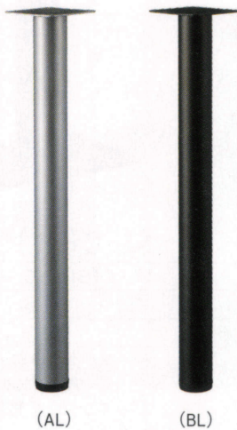
OL-E 脚部：60φパイプ（プレート付）・アジャスター付 高さ：680 天板サイズ：～W1500・～D800・～1200φ 1本 ¥6,800
